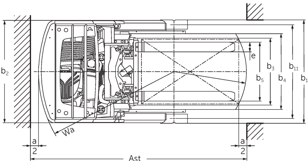
Dibujo técnico, ficha técnica ETV 216i
